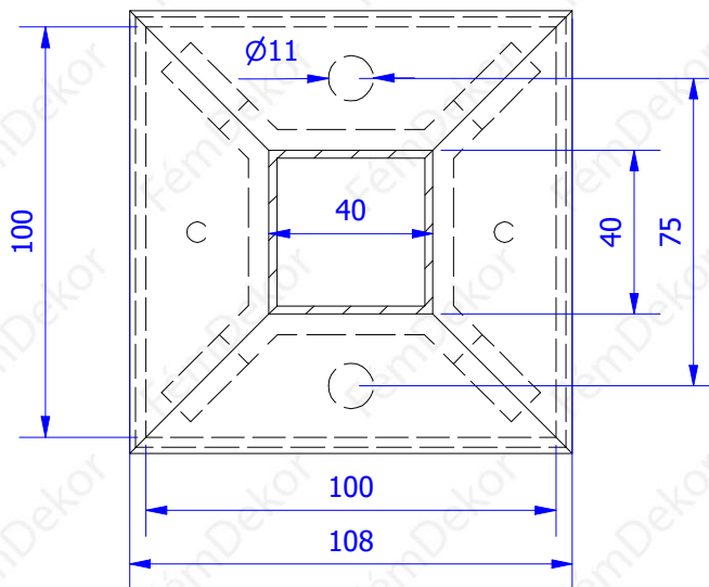
D-D ( 1 : 2 )
