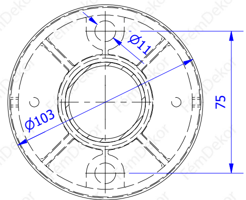
B-B ( 1 : 2 )
