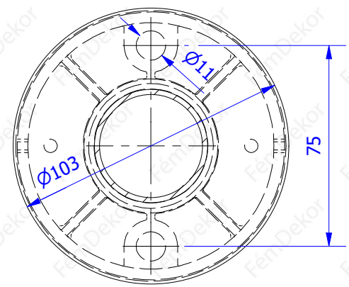
B-B ( 1 : 2 )
